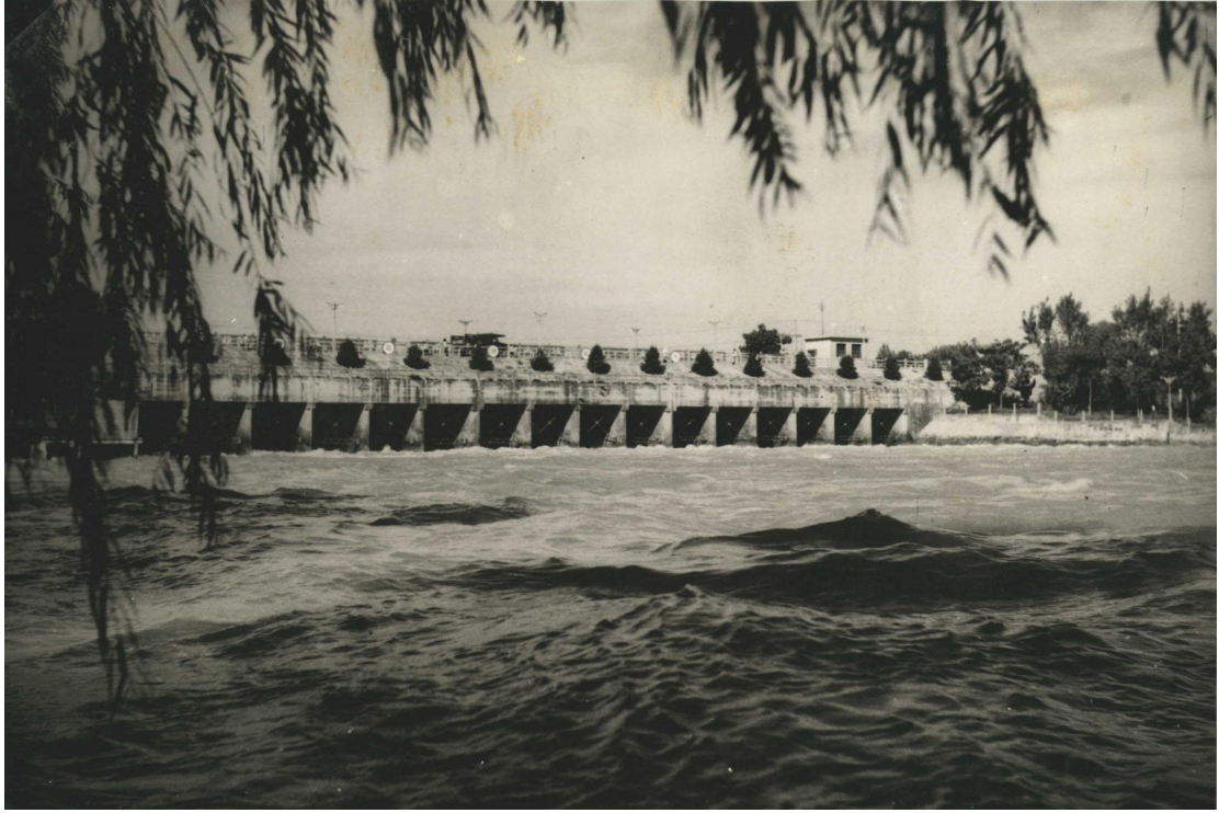
1978年，苏北灌溉总渠上的渠首闸，既能灌溉又能分洪，淮安市档案馆藏，档号：D018-1978-003-0027-0018
